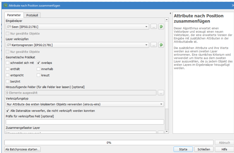
Abbildung 9. Räumliches Abfragefenster von QGIS
